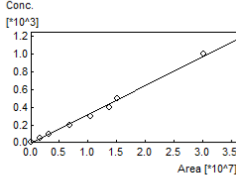
Şekil 2.3 Kalibrasyon grafiği
