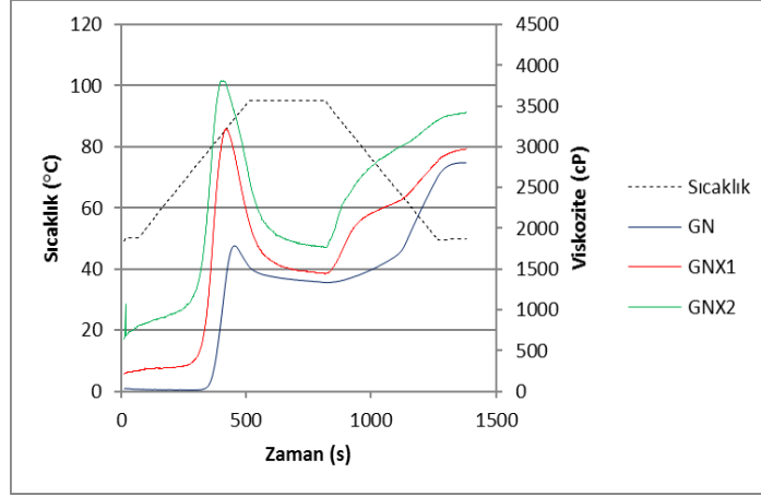
Şekil 4. 5 Gölevezi nişastası - ksantan gum karışımına ait jelleşme grafiği
