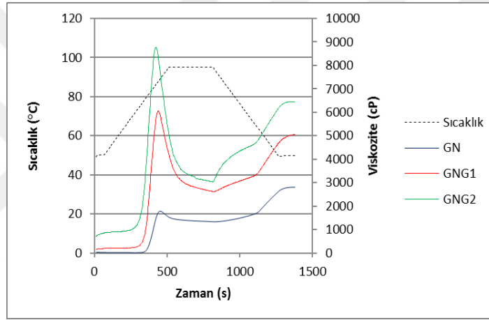
Şekil 4. 6 Gölevezi nişastası - guar gum karışımına ait jelleşme grafiği
