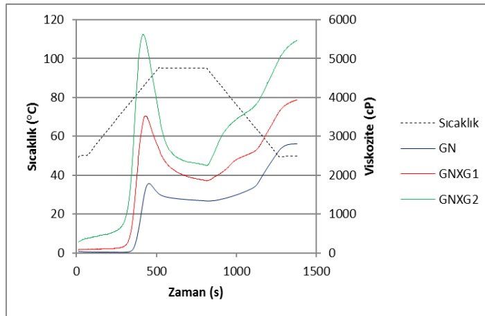
Şekil 4. 7 Gölevezi nişastası - ksantan gum- guar gum karışımına ait jelleşme grafiği
