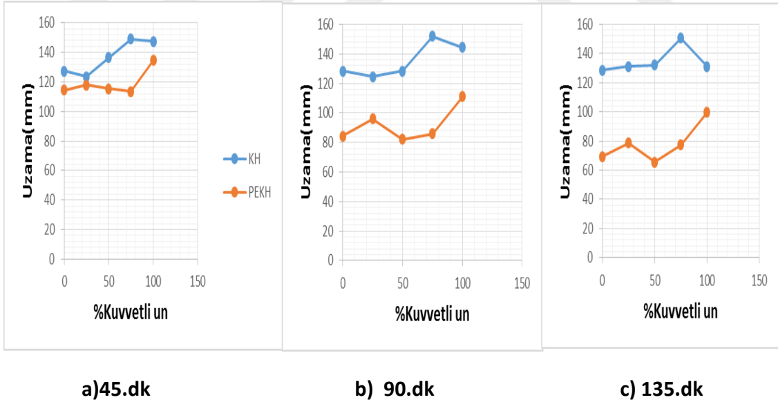
Şekil 4. 8 Pelemer ekstraktı katkılı un ile katkısız unun yüzdesel kuvvetli un artışına bağlı olarak uzama grafiği
