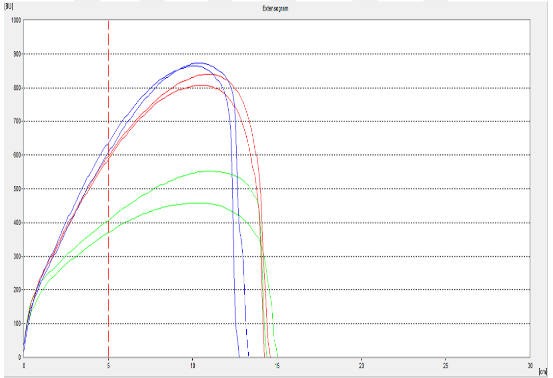
%100 kuvvetli un hamur ekstensograf grafiği
